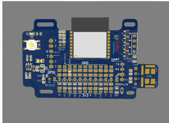
LEDFLY Wifi/Bluetooth Haberleşme Modülü
